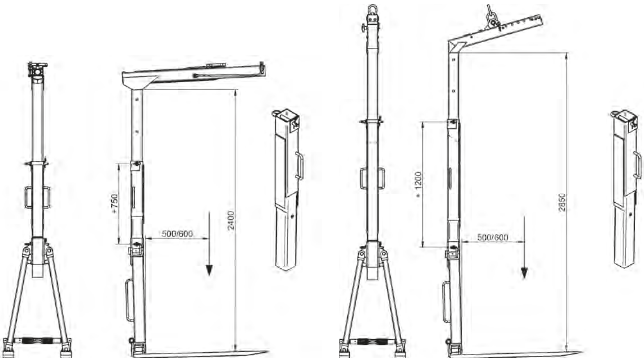
Verlängerung um 750 mm mit KM 401 H (ohne Drehmotor)
