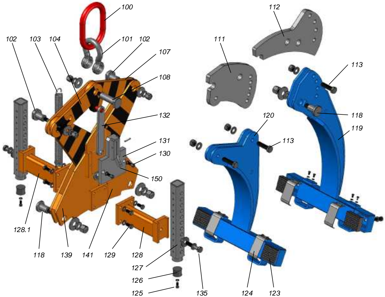
Arm Typ I – 50
